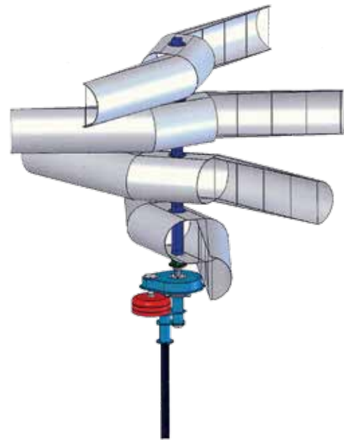
001269179-0001; vēja ģenerators; Nikolajs KUĻEŠOVS
